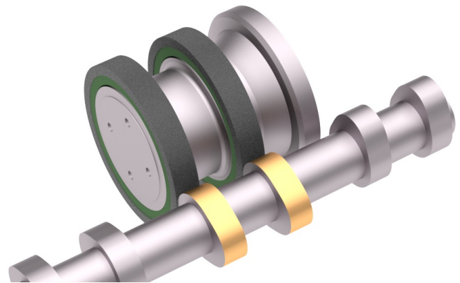
Schleifprozess: Unrundsleifen
